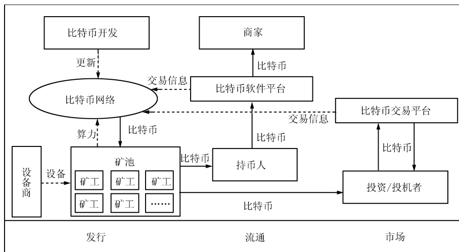
图 1 比特币生态圈 Fig. 1 The Bitcoin ecosystem
